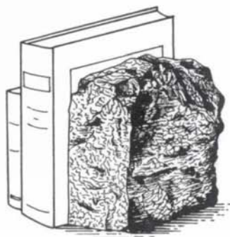
Feldspar
