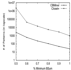
Fig. 10. # Patt. ( sports ).
