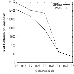
Fig. 8. # Patt. ( T40I10D100K ).
