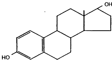
ESTRADIOL
