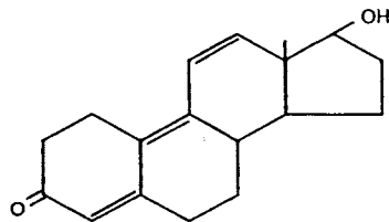
TRENBOLONE
