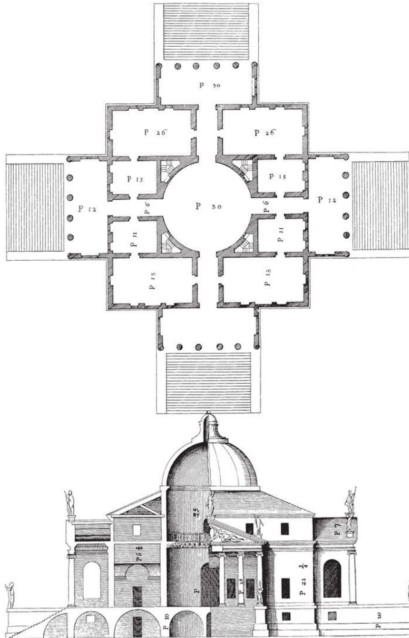
9. Andrea Palladio, Villa Rotonda, Vicenza, 1566 (Berzal, Javier 9 )
