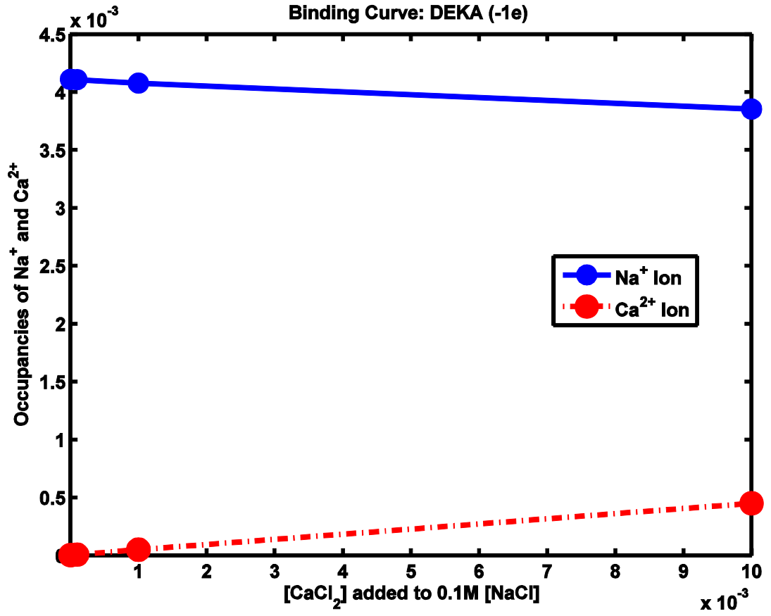
Fig. 3 Sodium (DEKA) channel
